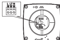
Podłączenie wentylatora 100/125/150 T, TH, VT, VTH
