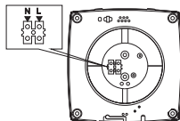
Podłączenie wentylatora 100/125/150
