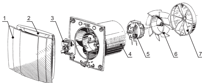
rys.1. 1-front, 2-pokrywa, 3-uk³ad steruj¹cy 4- korpus, 5- silnik elektryczny, 6- œmig³o/wirnik, 7- zawór zwrotny
